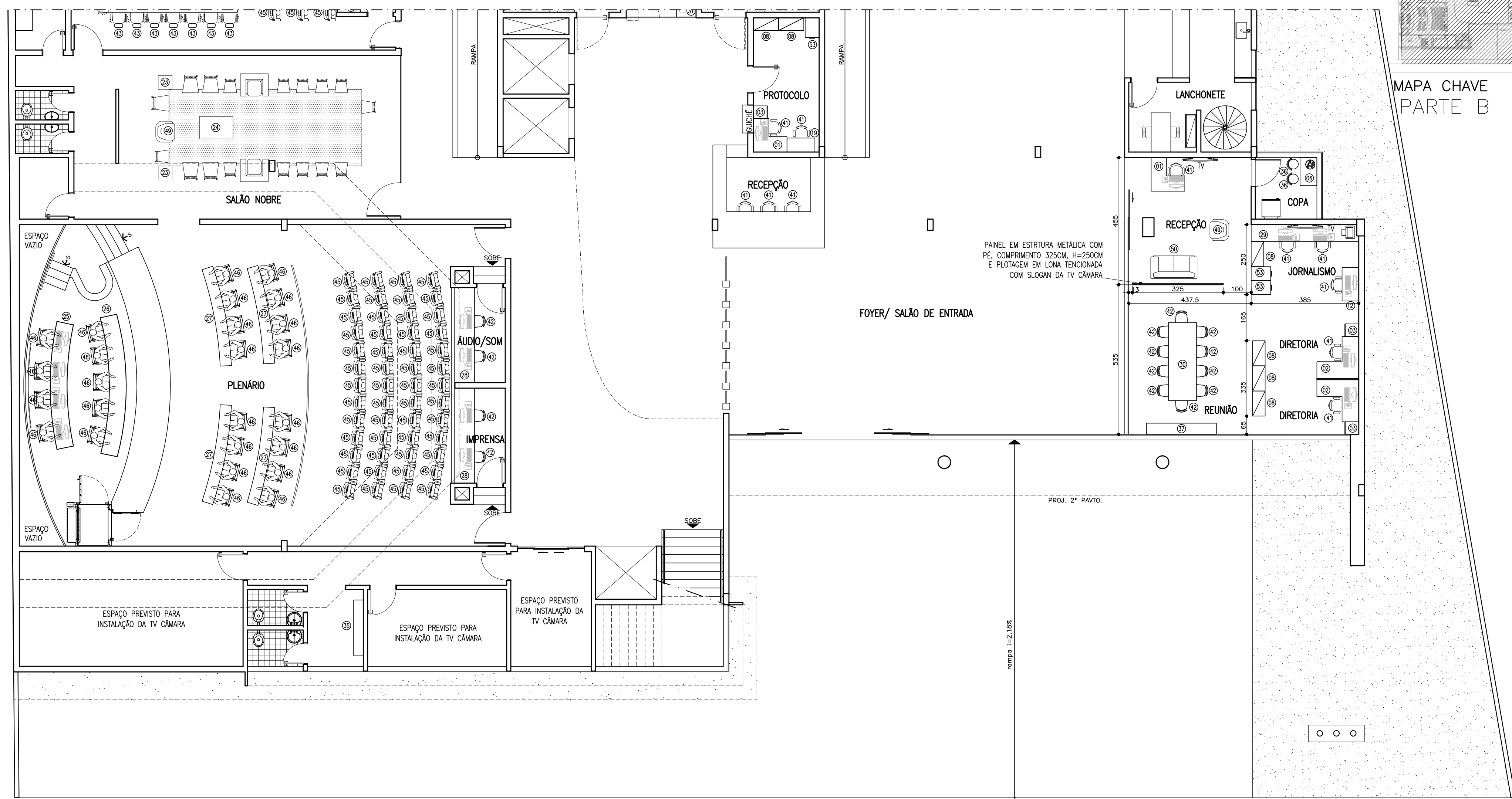
PLANTA TÉRREO escala 1:100
