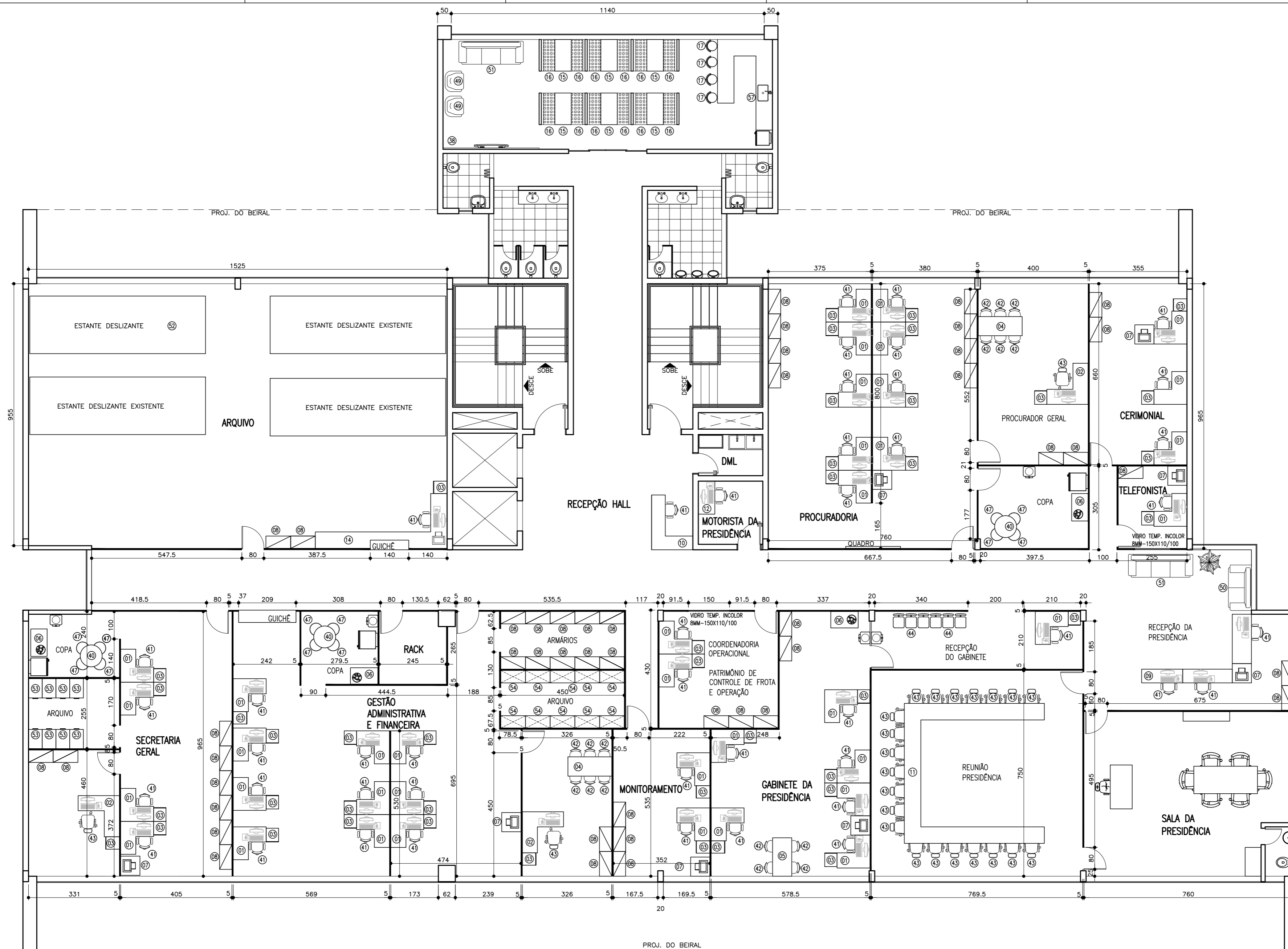
PLANTA 3º PAVIMENTO escala 1:100
